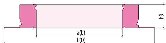
XRD XRD/W
